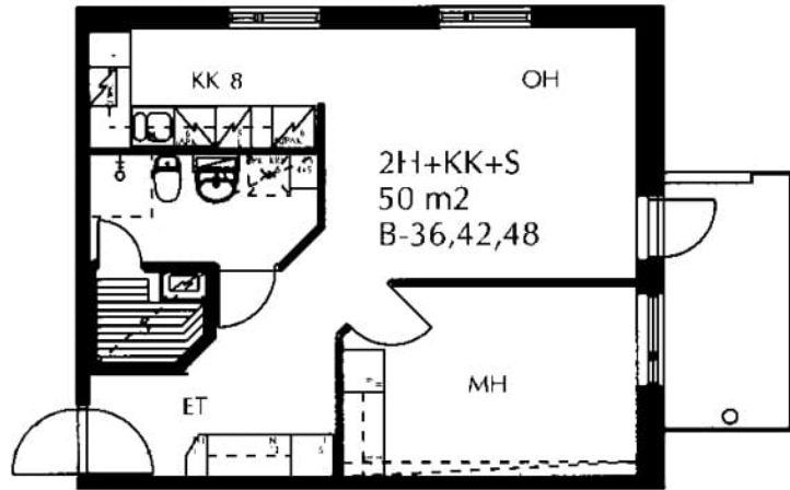
Krakantie 2B B 48 / pohjakuva Ei mittakaavassa
