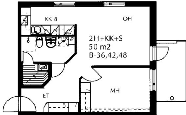
Krakantie 2B B 42 / pohjakuva
