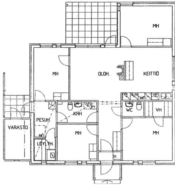
Matarinpolku 919 / pohjakuva Not in scale
