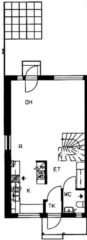
Kehäkukantie 44 C 5 / pohjakuva 1. kerros Ei mittakaavassa
