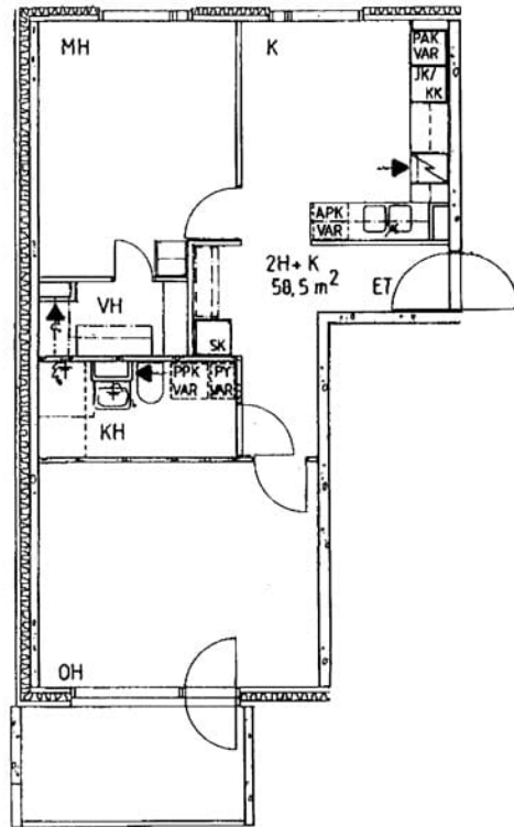
Vasamakatu 10 B 12 / pohjakuva Ei mittakaavassa
