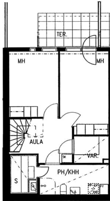
Sienitie 47 A 1 / pohjakuva 1. kerros
