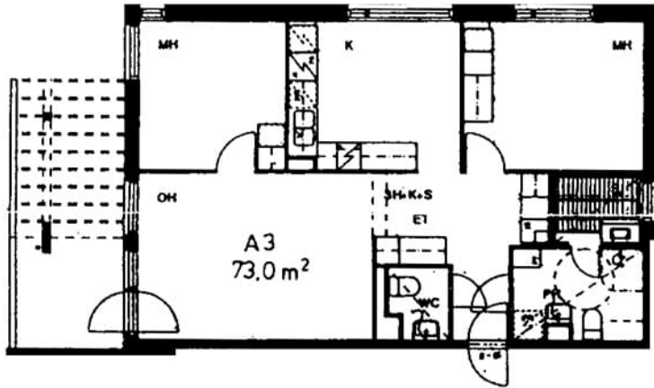
Kivikonkaari 7 A 3 / pohjakuva Ei mittakaavassa
