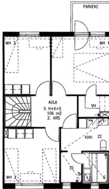
Sorvankaari 6 A 3 / pohjakuva 2.kerros Ei mittakaavassa
