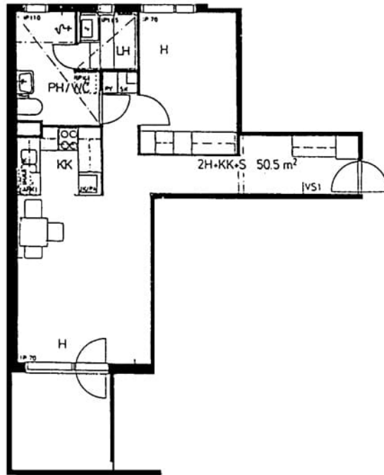
Albergan Esplanadi 4 A 7 / pohjakuva Ei mittakaavassa
