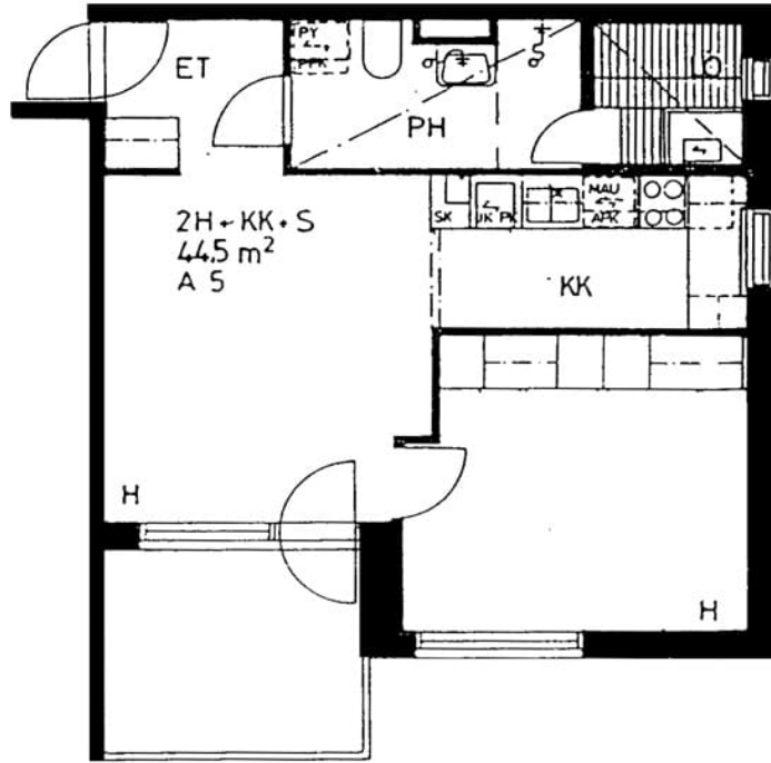
Iso-Hollonkuja 8 A 1 / pohjakuva Ei mittakaavassa
