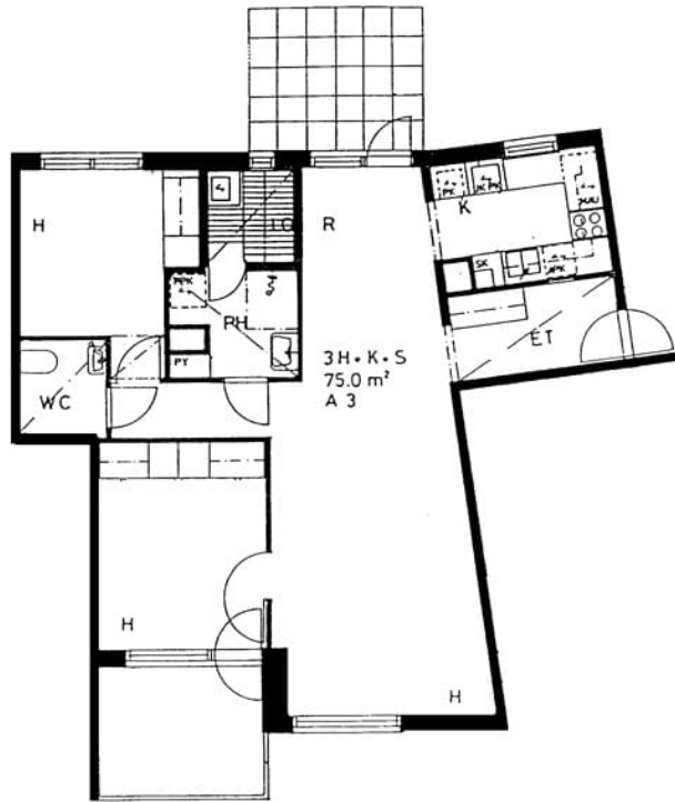
Iso-Hollonkuja 8 A 11 / pohjakuva Not in scale
