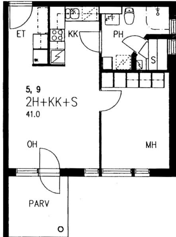
Papulintie 9 A 5 / pohjakuva Not in scale
