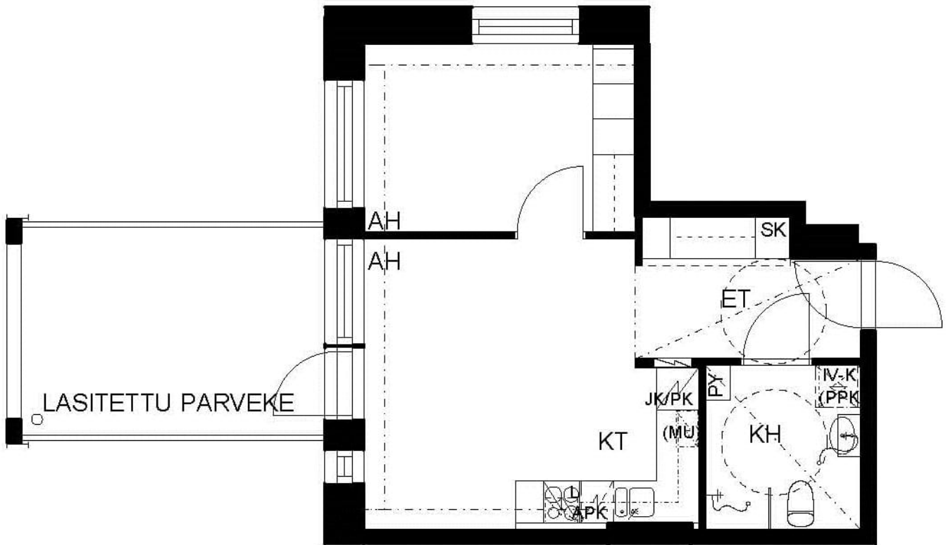
Ulrikankuja 20 A 1 / pohjakuva Ei mittakaavassa
