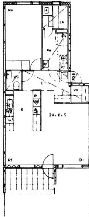
Sinettikuja 4 B 15 / Pohjakuva Not in scale
