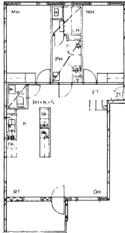
Sinettikuja 4 B 21 / Pohjakuva Ei mittakaavassa
