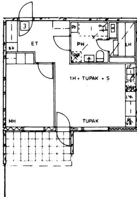
Sinettikuja 4 A 11 / Pohjakuva
