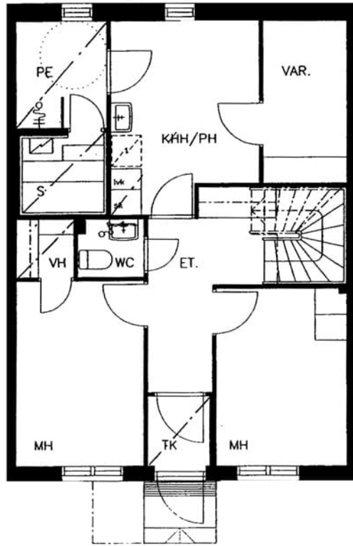
Kokkokalliontie 5 E 5 / pohjakuva 1. kerros
