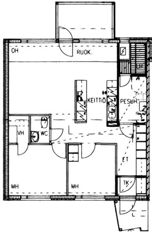
Penttilänkatu 3 B 10 / pohjakuva Ei mittakaavassa
