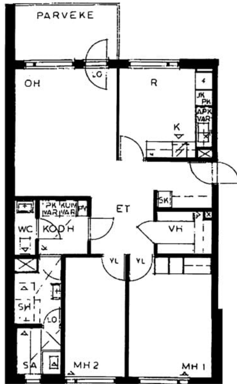
Keilakuja 2 B 14 / pohjakuva Not in scale
