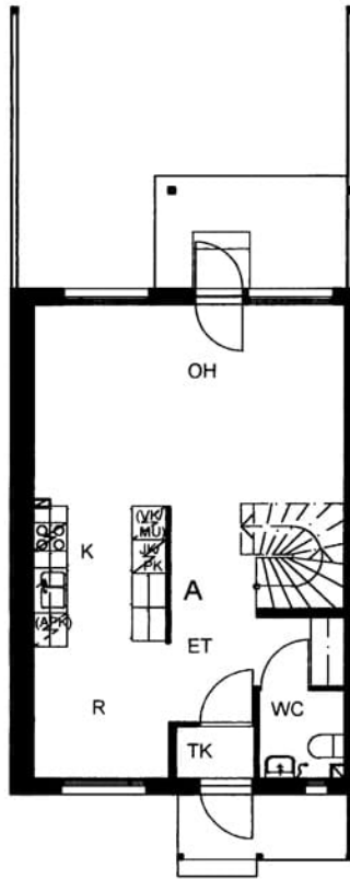
Vartiokuva 2 A 1 / pohjakuva 1. kerros Ei mittakaavassa
