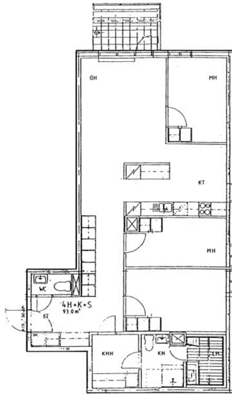
Saimaankatu 58 B A 29 / pohjakuva Not in scale
