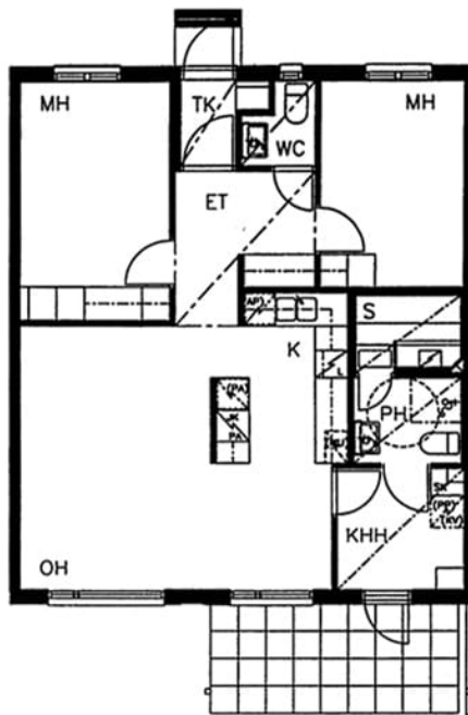
Pesäpolku 3 C 17 / pohjakuva Not in scale
