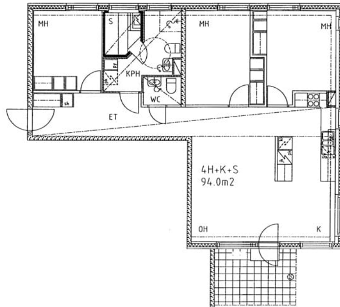
Huvilakatu 20 A 5 / pohjakuva
