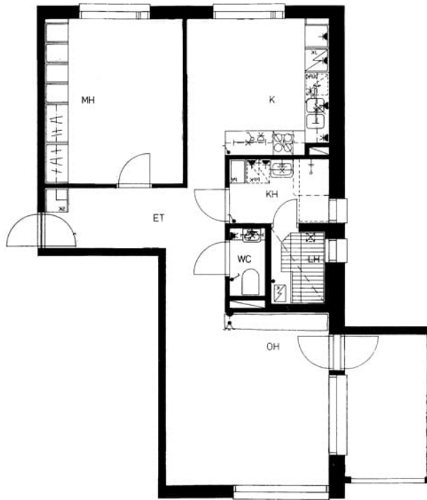
Snellmanintie 9 A 8 / pohjakuva Not in scale
