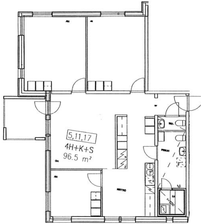
Kangastuvankatu 8 A 17 / pohjakuva Ei mittakaavassa
