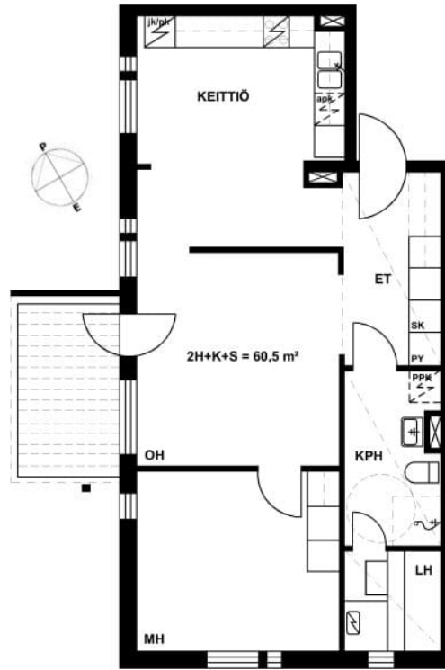
Läntinen Kanavatie 31 As 2 / Pohjakuva Ei mittakaavassa
