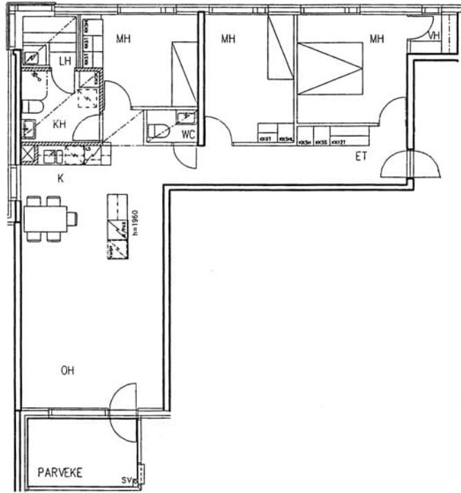
Satamakatu 23 B 27 / pohjakuva Not in scale
