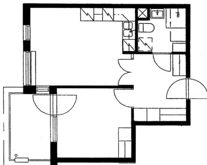
Ounasvaarantie 7 A 5 / pohjakuva
