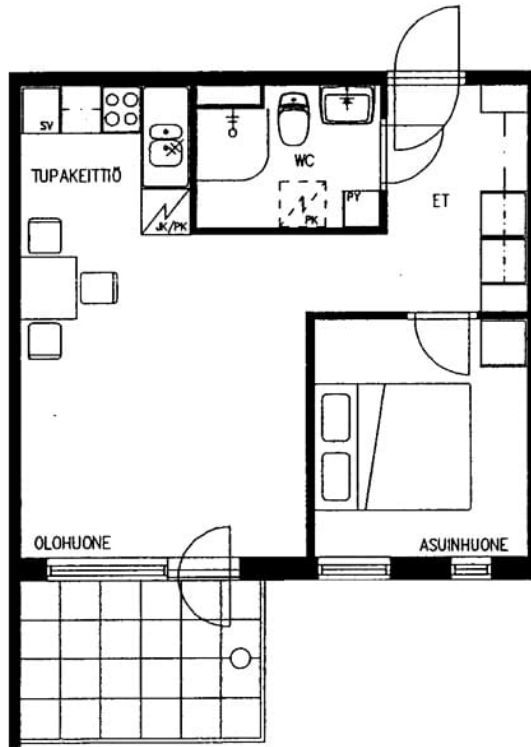
Hovinkatu 5 A 12 / pohjakuva
