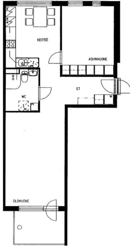
Hovinkatu 5 A 11 / pohjakuva Not in scale
