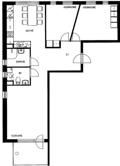
Hovinkatu 5 B 28 / pohjakuva Not in scale
