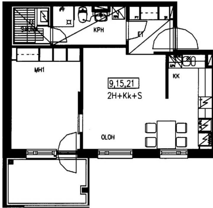
Rantakatu 16 As 9 / pohjakuva
