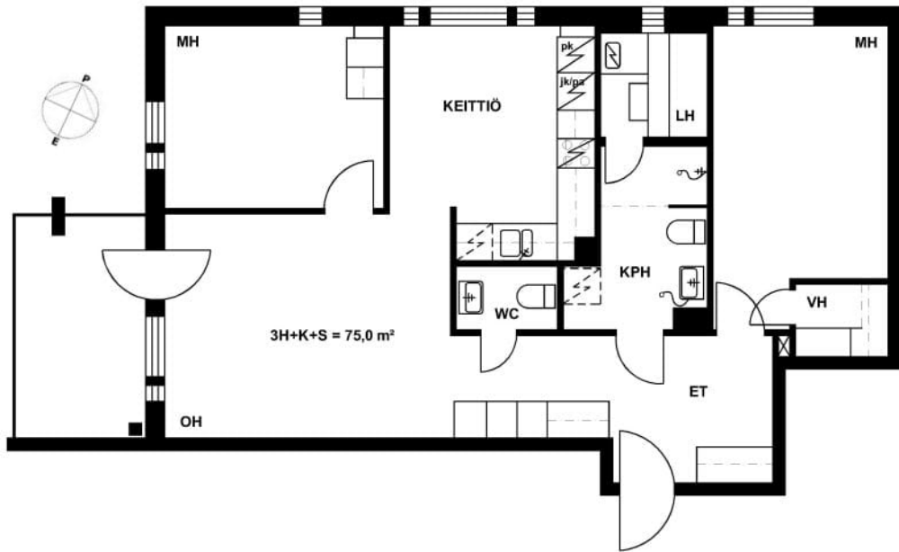
Pikisaarenkatu 41 A 30 / Pohjakuva Ei mittakaavassa
