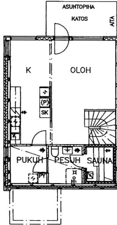
Taavinharju 16 G 14 / pohjakuva 1.kerros Ei mittakaavassa
