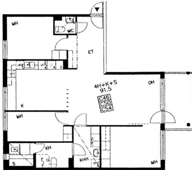
Tapulikaupungintie 15 C 50 / pohjakuva
