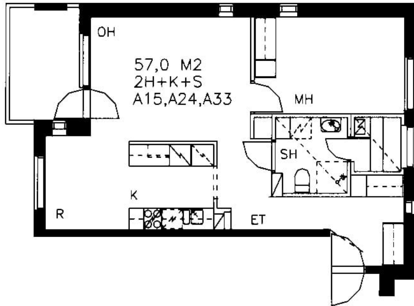
Karsikkokuja 6 A 33 / pohjakuva Ei mittakaavassa
