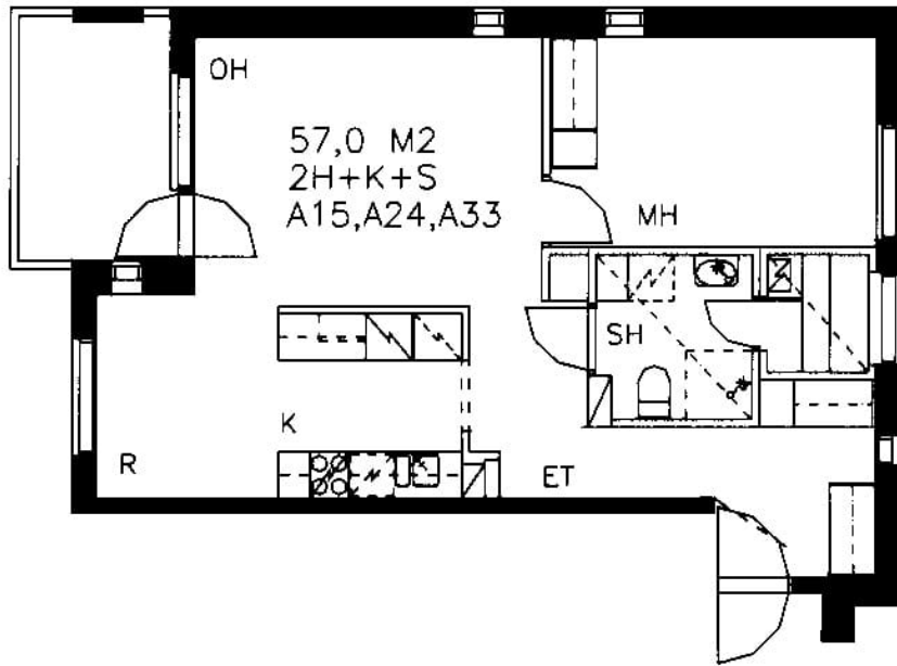
Karsikkokuja 6 A 15 / pohjakuva Not in scale
