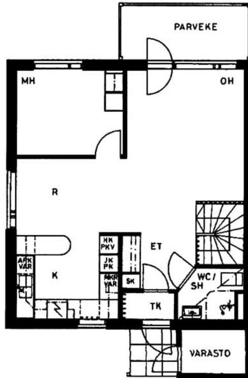
Nousutie 18 A1 / pohjakuva 2. kerros Not in scale
