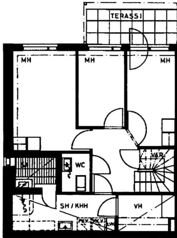
Nousutie 18 A 1 / pohjakuva 1. kerros Not in scale
