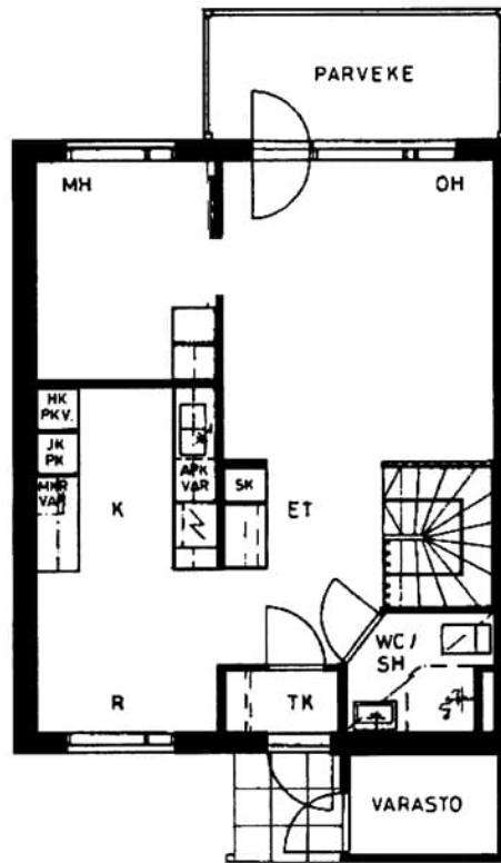
Nousutie 18 C 5 / pohjakuva 2. kerros Ei mittakaavassa
