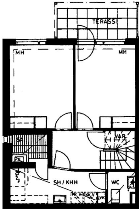
Nousutie 18 C 5 / pohjakuva 1. kerros Ei mittakaavassa
