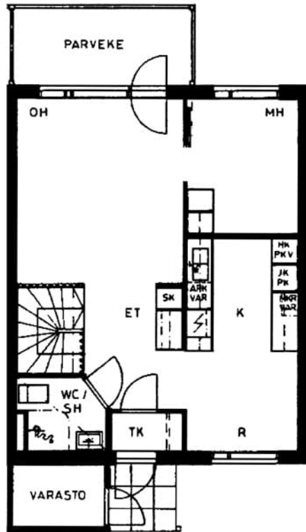
Nousutie 18 C 6 / pohjakuva 2. kerros Ei mittakaavassa
