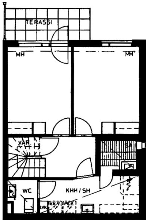
Nousutie 18 C 6 / pohjakuva 1. kerros Ei mittakaavassa
