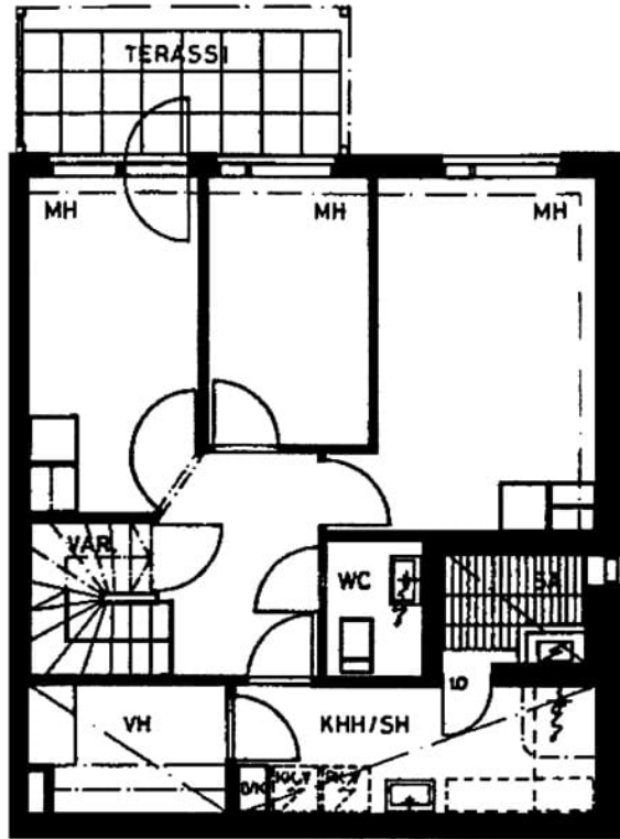
Nousutie 18 B 4 / pohjakuva 1. kerros Not in scale
