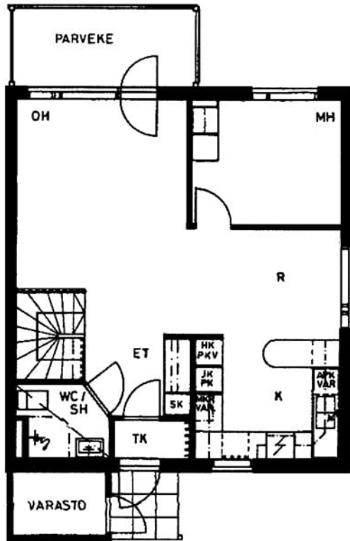
Nousutie 18 B 4 / pohjakuva 2. kerros Not in scale
