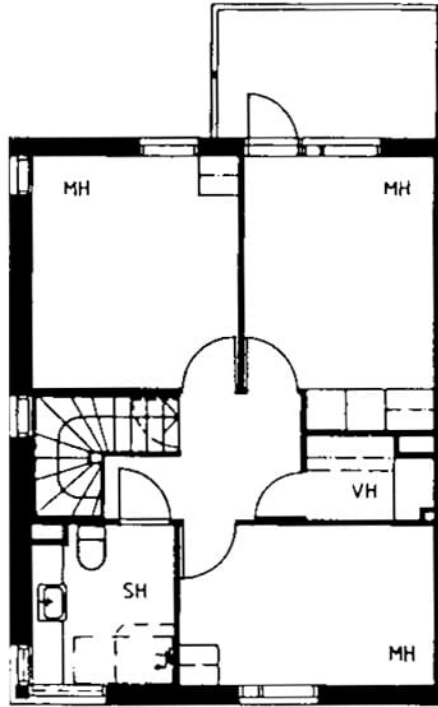
Ramsinniementie 5 G 34 / pohjakuva 3.kerros Ei mittakaavassa
