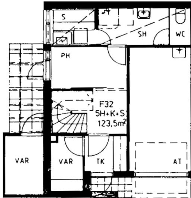
Ramsinniementie 5 G 34 / pohjakuva 1.kerros Ei mittakaavassa
