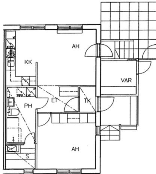
Tikkurikuja 10-12 F 6 / pohjakuva
