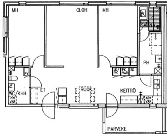
Sarvikatu 6 A 11 / pohjakuva
