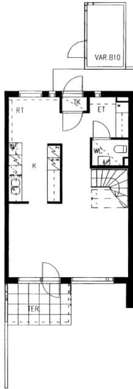
Kaivantokuja 2 B 10 / pohjakuva 1. kerros Not in scale
