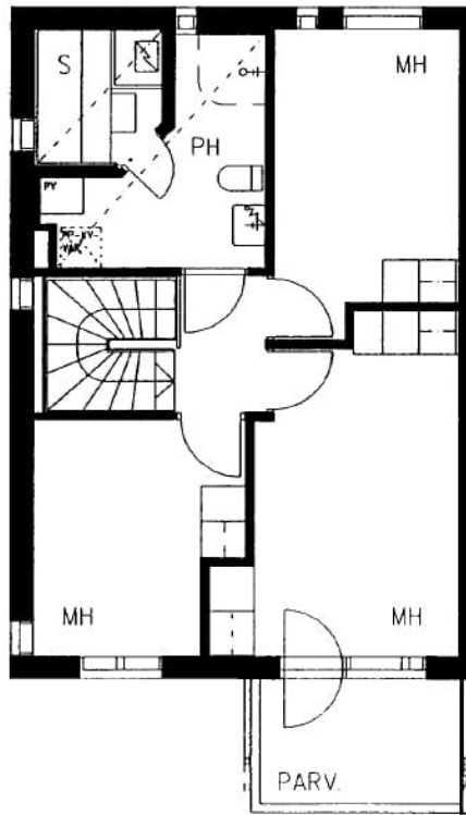
Kaivantokuja 2 B 11 / pohjakuva 2. kerros
