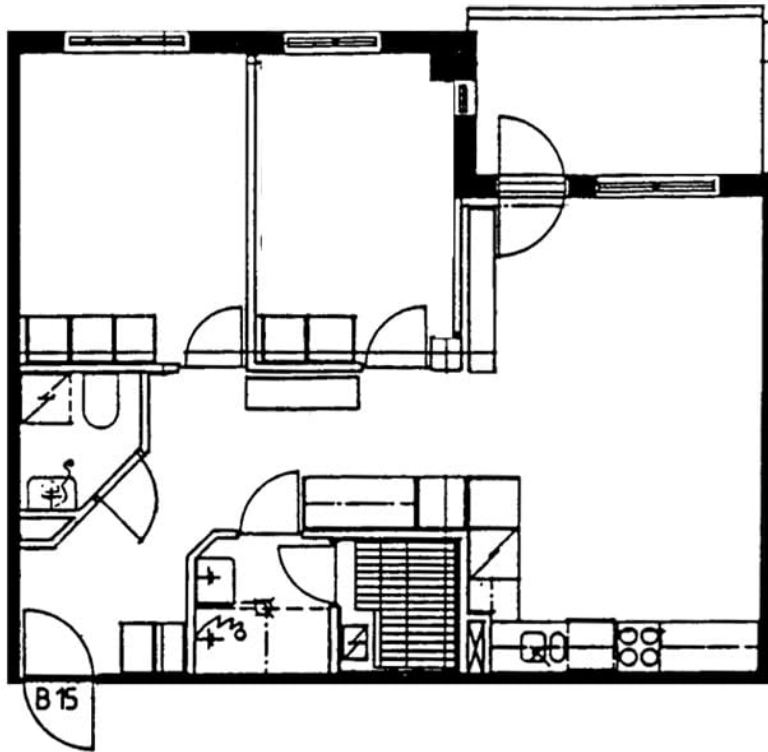
Uusikatu 43 A 4 / pohjakuva Not in scale
