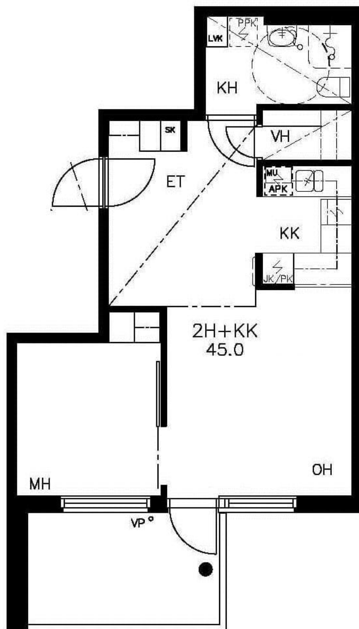
Huvilinnanmäki 2 A 44 / pohjakuva
